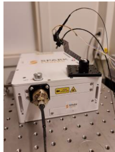
ミンスコープに接続された ALCOR 920-Mini2P の写真 (Kavli研究所, NTNU “Mini2Pチーム”提供)
