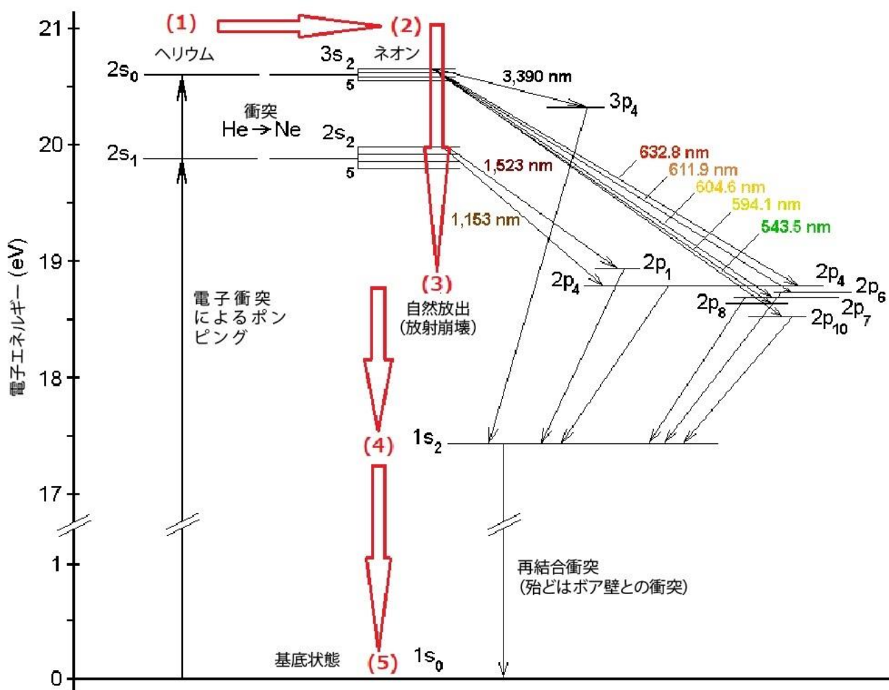
HeNe励起と発振過程
