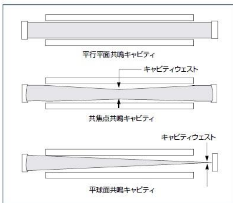
レーザーキャビティのタイプ
